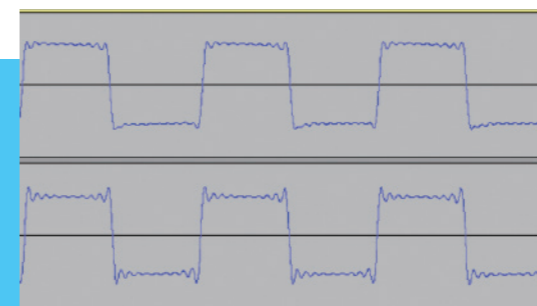
訊號輸出(上)耳擴輸出(下) 1kHz方波表現
